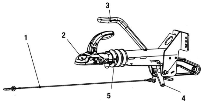
Kuva 2: jarrupää (työntöjarru)
